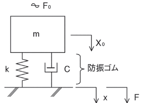
図-1 防振のモデル
