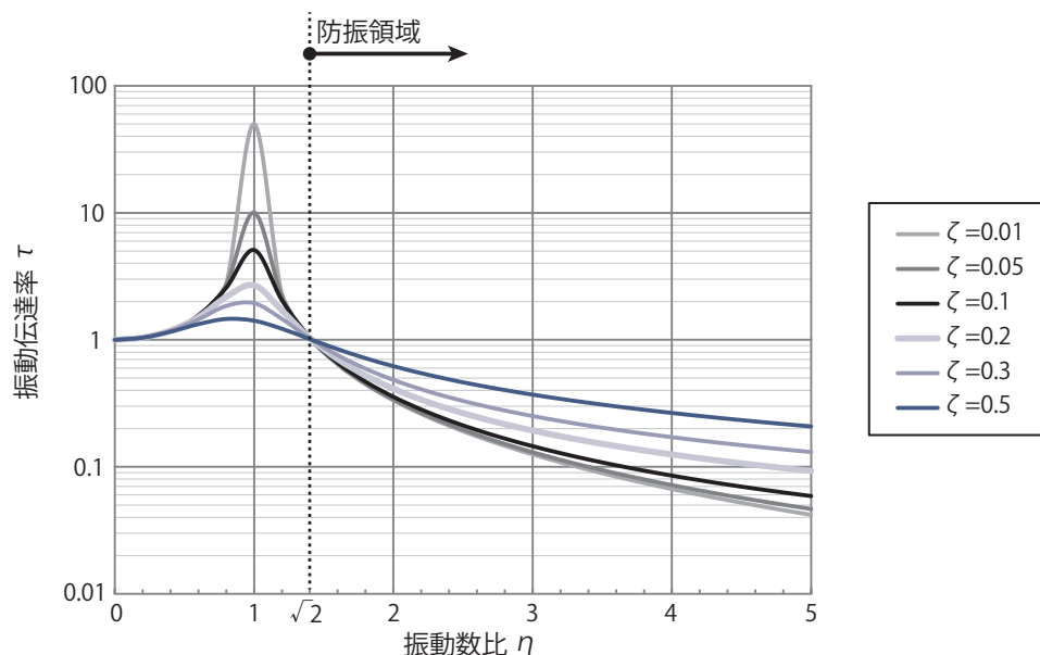
図-2 振動伝達率と減衰比の関係
